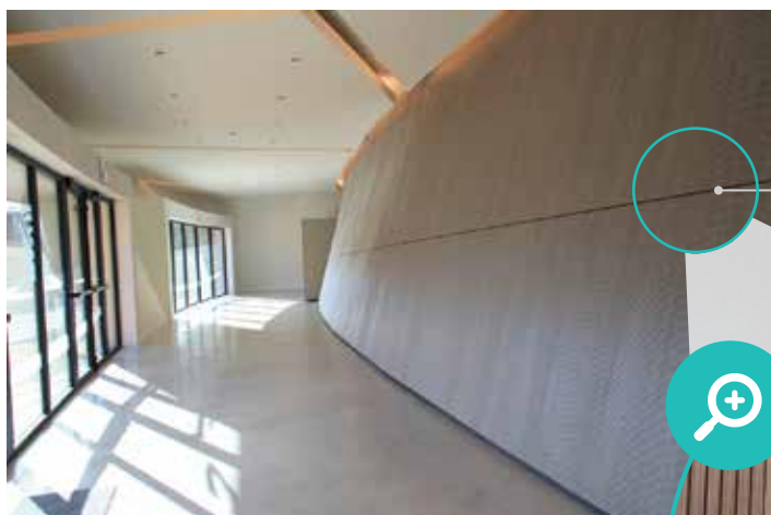
fig 17. Kopse montage gegroefde panelen of planchetten: werken met schaduwvoeg
